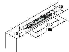
Routing dimension Kích thước khoan cắt
