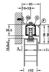
Wall installation with clip panel Treo tường với nắp che
