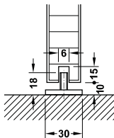
Floor guide without guide track in door leaf Dẫn hướng sàn không có thanh dẫn hướng gắn cửa
