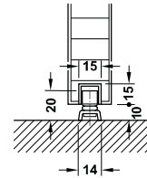
Floor guide with U-shaped guide track in door leaf and floor guide roller Dẫn hướng sàn có bánh xe và ray chữ U gắn cửa
