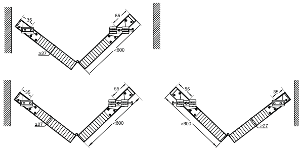
Top view installation Mặt chiếu bằng
